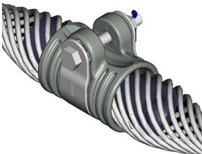
GRAPA DE REMATE A COMPRESIÓN
